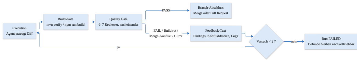
Abbildung 19.7.: Die Korrekturschleife als Regelkreis — Befunde werden zu Eingaben des nächsten Laufs
