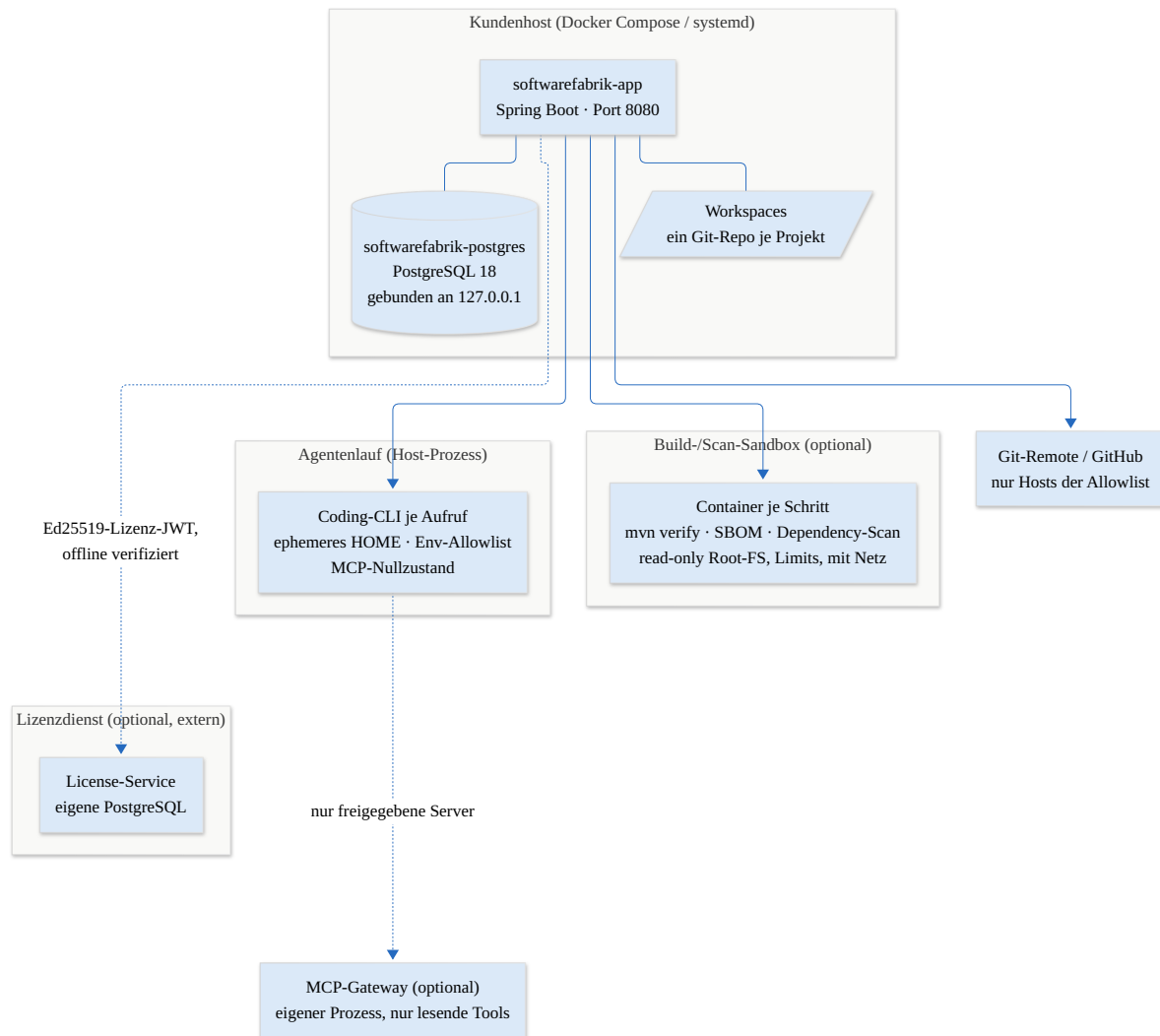
Abbildung 19.10.: Deployment-Sicht: ein Anwendungscontainer, eine Datenbank, optional getrennter Lizenz-Stack. Air-Gap-fähig
