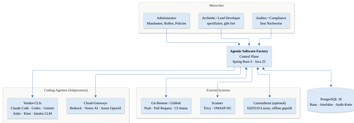
Abbildung 19.1.: Systemkontext der Agentic Software Factory: eine Control Plane zwischen Mensch, Coding-Agenten und Zielrepository
