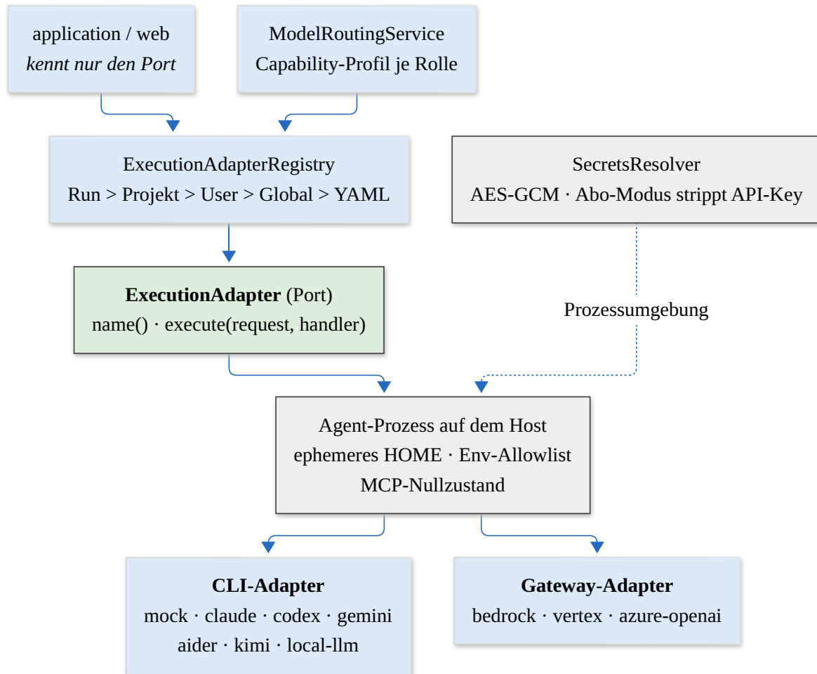
Abbildung 19.8.: Vendor-Neutralität durch einen Port: Application- und Web-Schicht kennen ausschließlich den ExecutionAdapter (ArchUnit-erzwungen)
