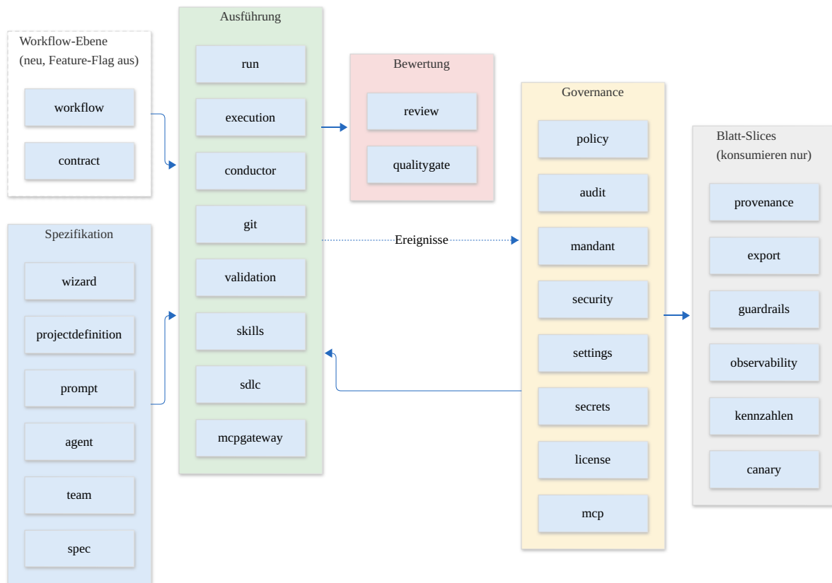
Abbildung 19.3.: Fachliche Slices der Fabrik, gruppiert nach Aufgabe. Blatt-Slices (provenance, export, guardrails, observability, kennzahlen, canary) werden von keinem Kern-Slice konsumiert; die technischen Querschnittspakete common und web sind nicht dargestellt
